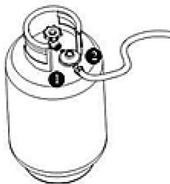
Punctul în care se face testul de etanșeitate ① ②
